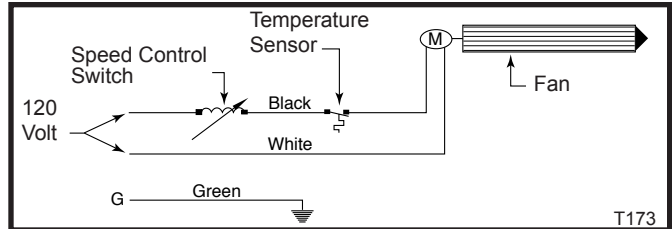
Fig. 36 Fan wiring diagram.
