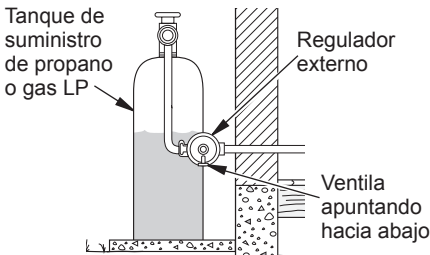
Figura 10 - Regulador externo con la ventila apuntando hacia abajo
