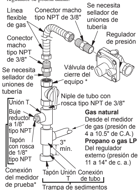
Figura 11 - Conexión de gas
