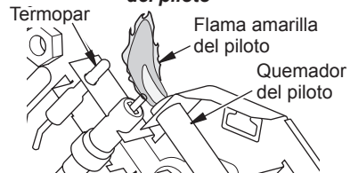
Figura 19 - Patrón incorrecto de la llama del piloto
